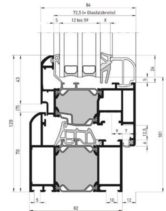
Schnittdarstellung BLECHER Alu W 72 RL
