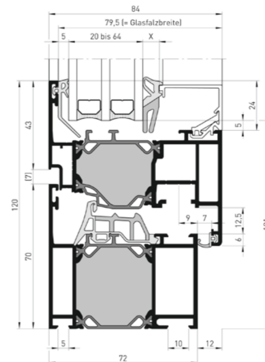
Schnittdarstellung BLECHER Alu W 72
